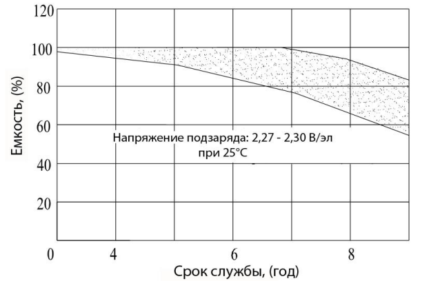
Срок службы в буферном режиме
